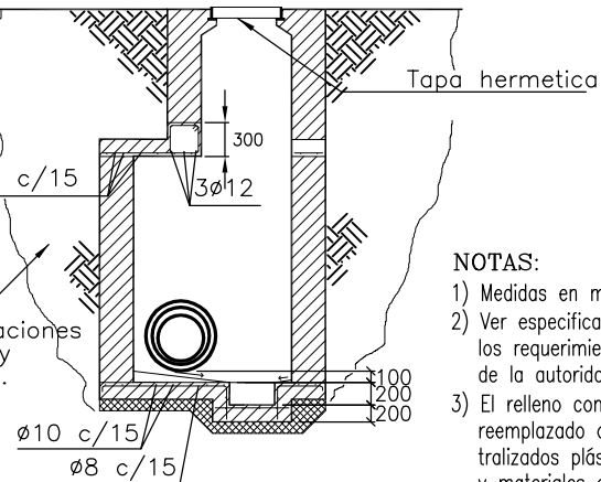
CORTE B-B
