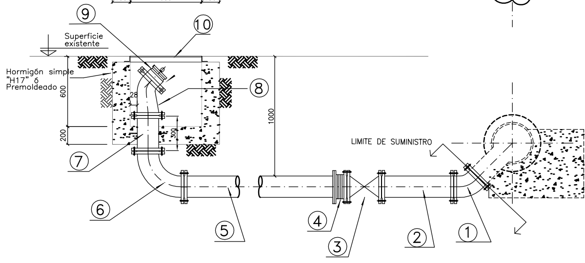
ELEVACION
