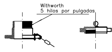
CORTE A-A
