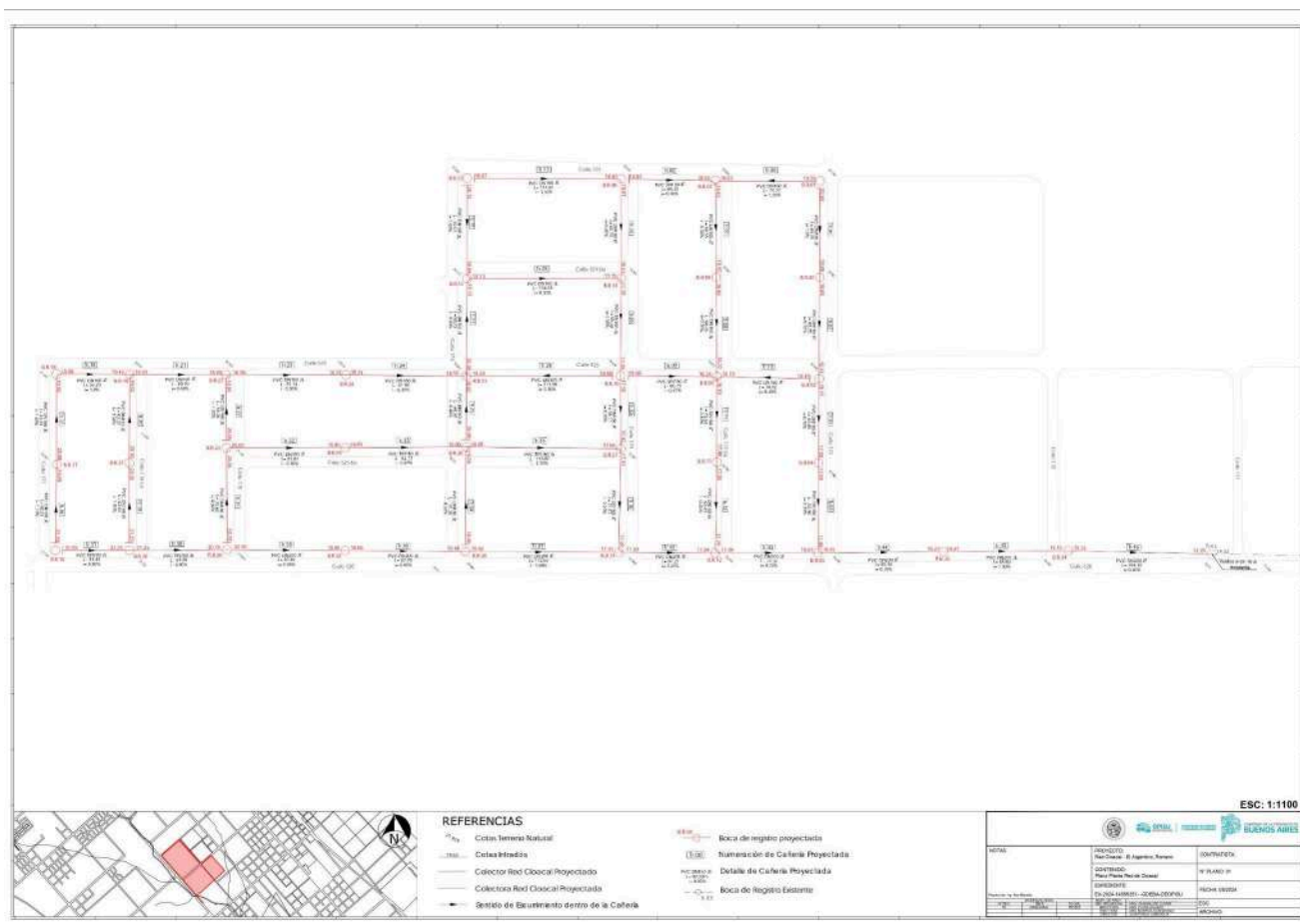
Figura N°1. Plano Red Cloacal. Fuente: Elaboración propia.
