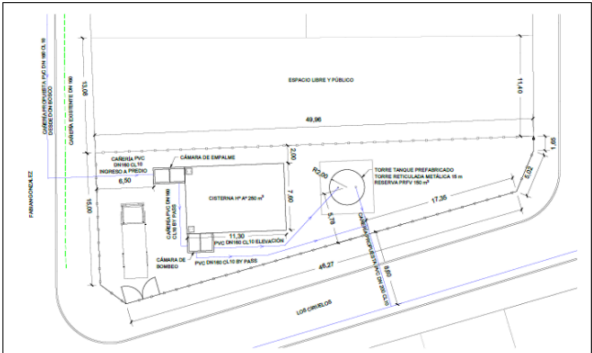
Figura N°3. Planta de predio tanque.
