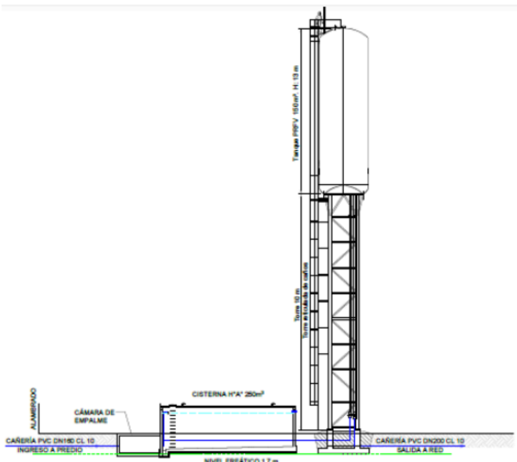
Figura N°4. Perfil de predio tanque.
